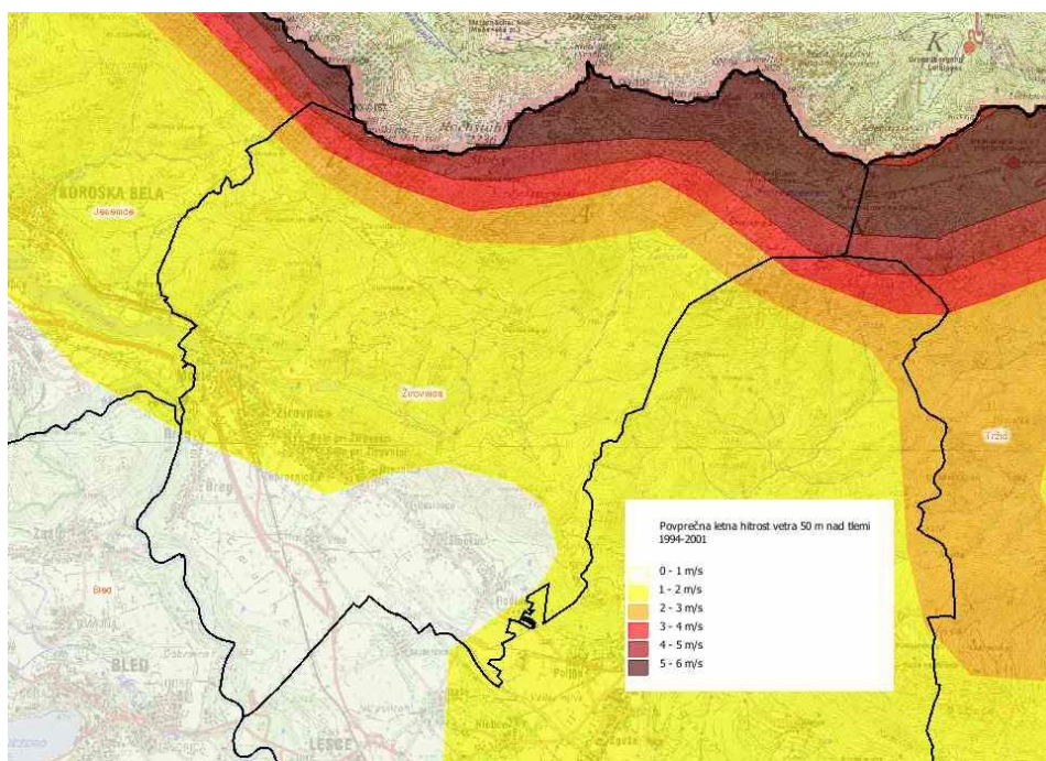
Slika 49: Povprečna letna hitrost vetra 50m na tlemi (1994-2001)
