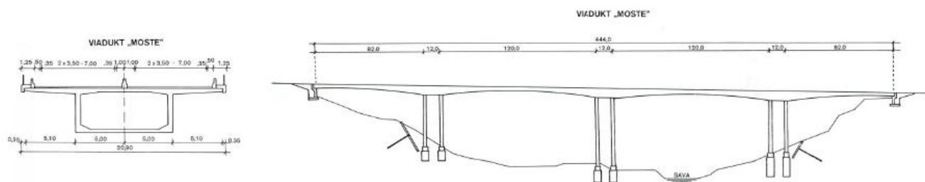
Slika 54: Viadukt Moste
