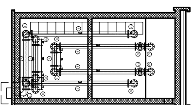
PREREZ 4-4
