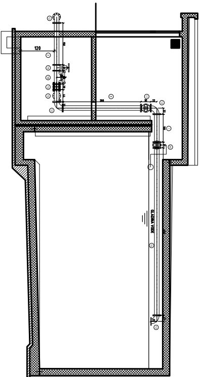
PREREZ 2-2 DOTOK
