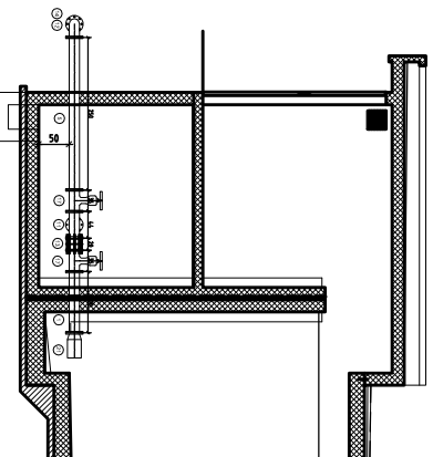
PREREZ 1-1 ODTOK
