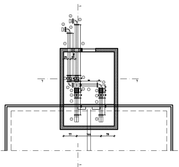
TLORIS 1-1 ODTOK
