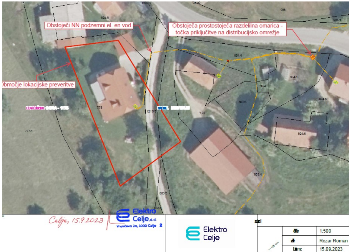
Slika 8: Prikaz elektro omrežja na območju LP; vir: Elektro Celje d.d.
