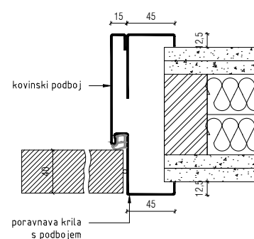
DETAJL PODBOJA
