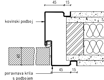
DETALJ PODBOJA
