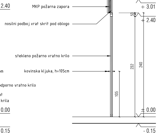
PREREZ
