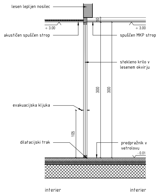
PREREZ
