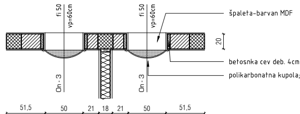
TLORIS
