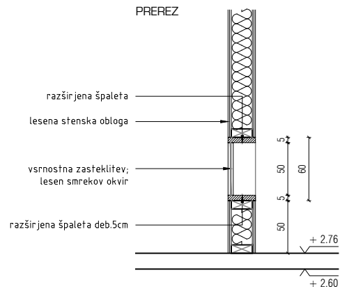
PREREZ
