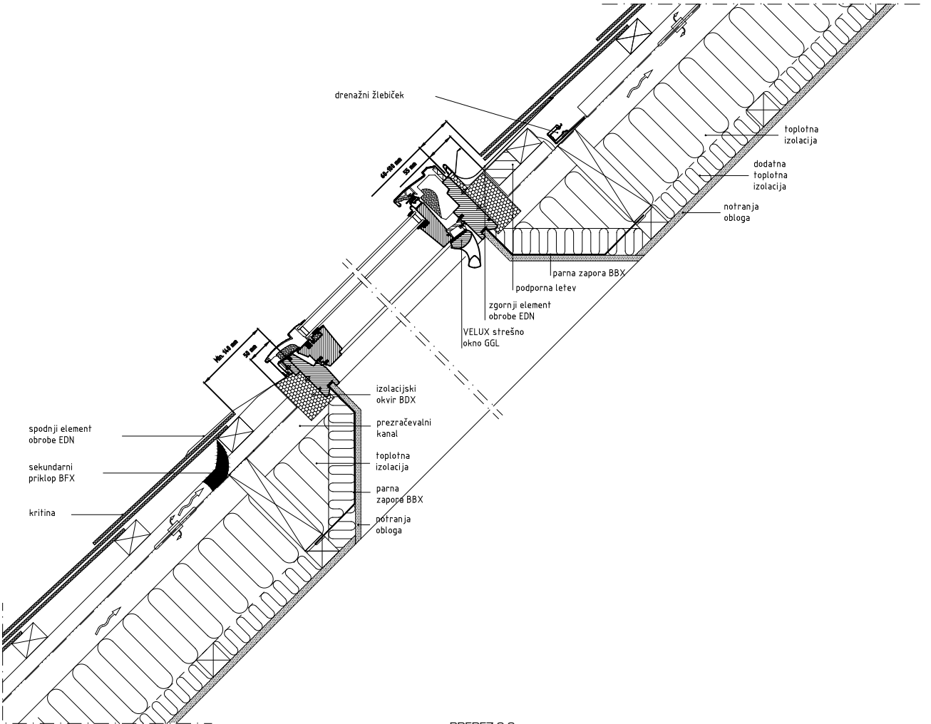
PREREZ 2-2
