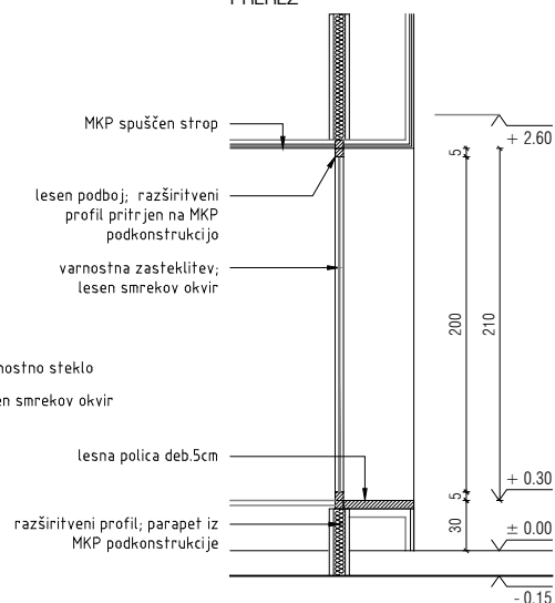
PREREZ
