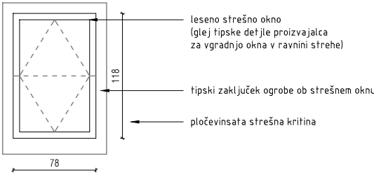
TLORIS
