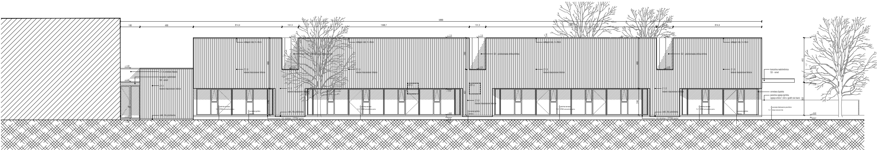
JUŽNA FASADA
