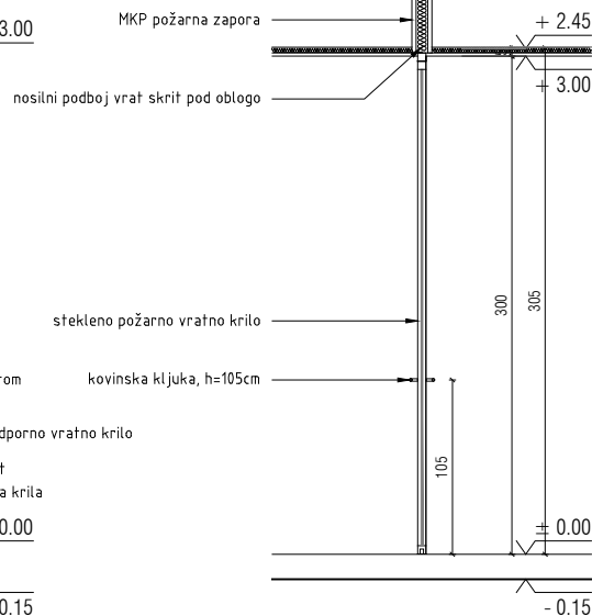
PREREZ
