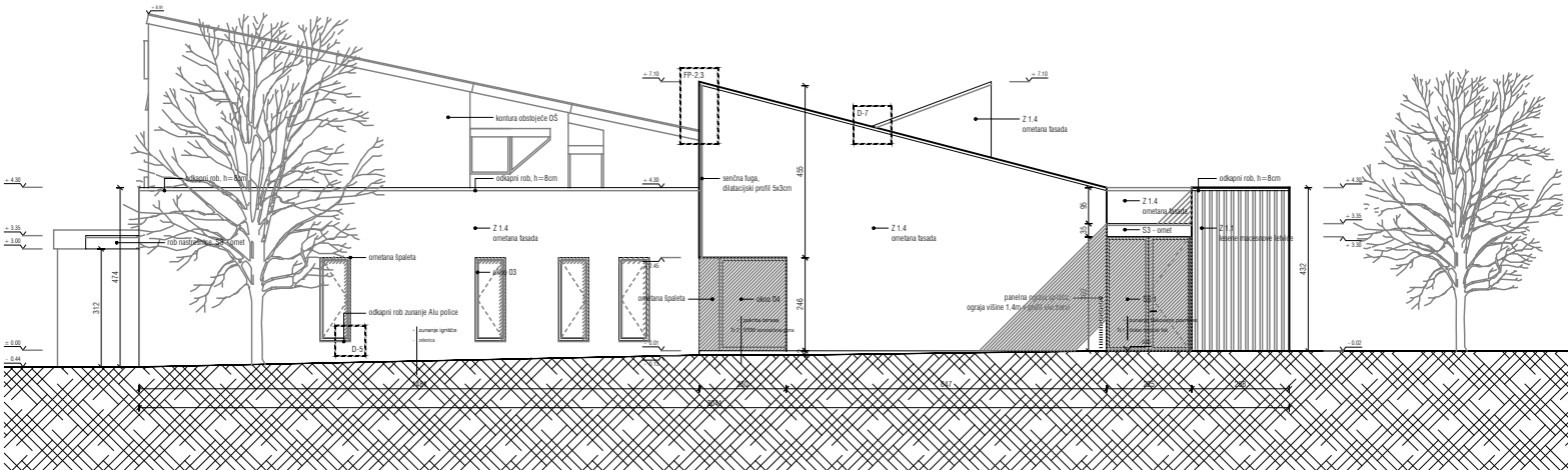
VZHODNA FASADA
