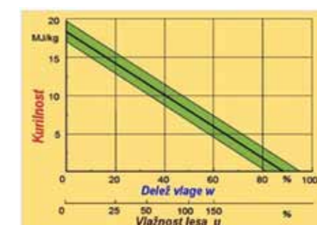
Slika 4: Odvisnost kurilnosti v MJ/kg od deleža vlage v drveh in vlažnosti drv. (vir: TFZ Bayern)
