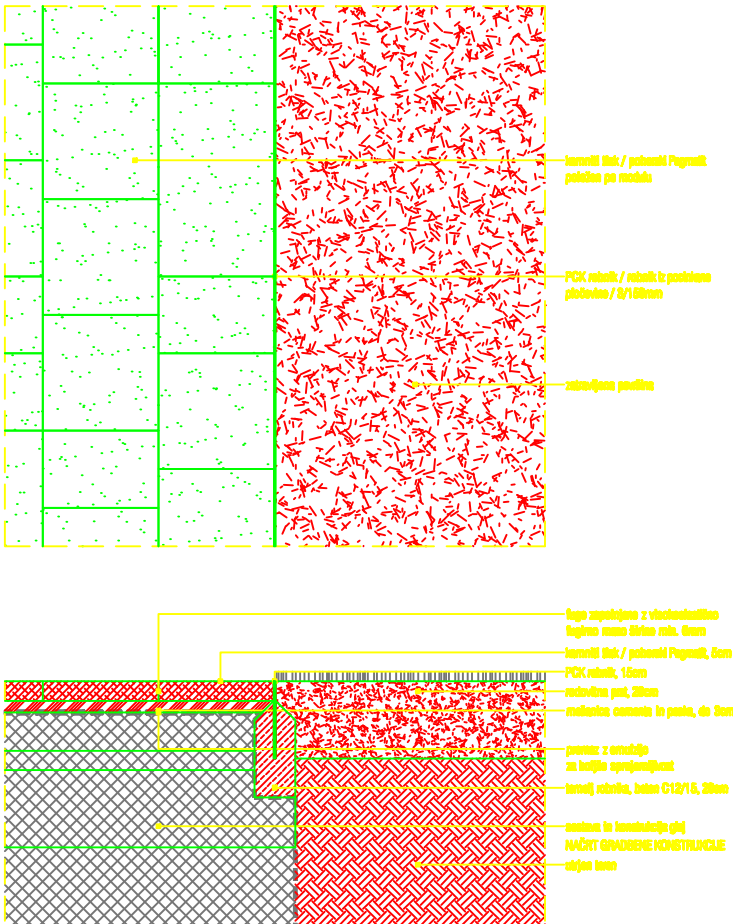
Detalji stika: kamniti tlak / PCK robnik / zatravljena površina
