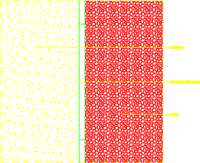
Detajl stika: drobljenec / AB robnik / prodec
