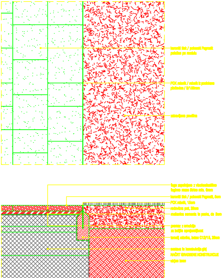
Detalji stika: kamniti tlak / PCK robnik / zatravljena površina
