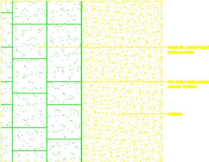
Detalji stika: kamniti tlak / PCK robnik / drobljenec
